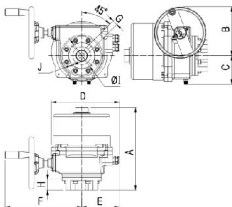
NOM-4...7A(B)-E / NOM-P4...7A(B)-E
