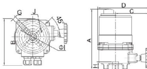
NOM-3A-E/ NOM-P3A-E
