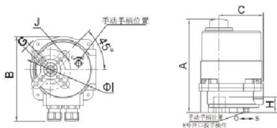
NOM-1...2A-E/ NOM-P1...2A-E
