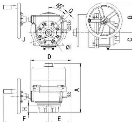
NOM-8A-E/ NOM-P8A-E
